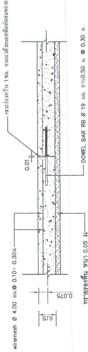
รูปขยายรอยต่อเพื่อการหดตัว (CONTRACTION JOINT)
